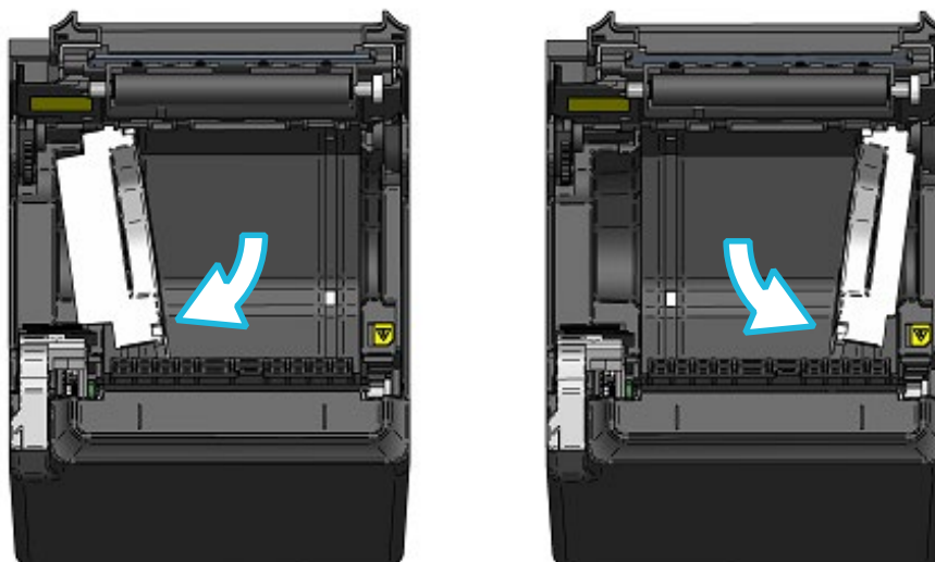
Illustration 14-2 Montage de la plaque de séparation (2)
