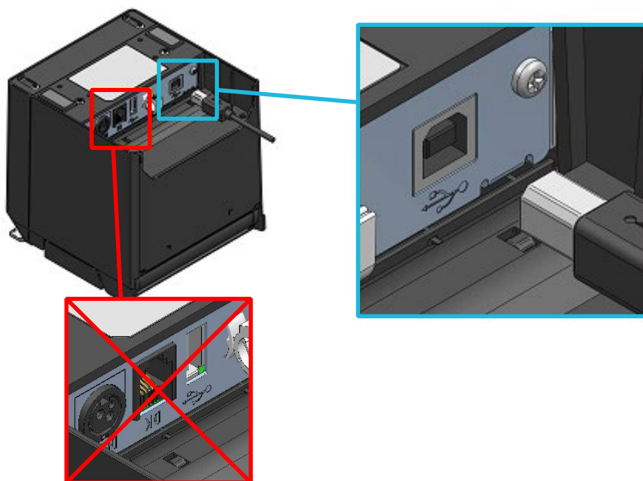
Illustration 12-1 Branchement du câble USB à l'imprimante
